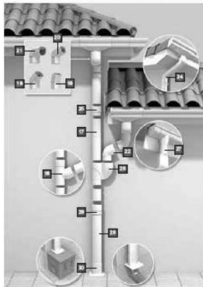
Rura spustowa Owacja TD 95 - 90 x 56 | TD 107 : 105x76
